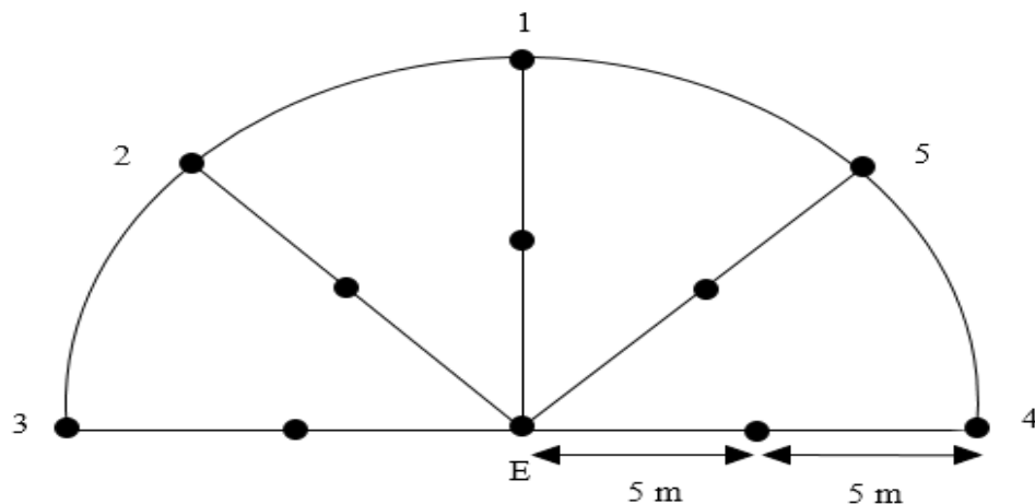
Gambar 6: Skema Pengukuran Tahanan Pengetanahan
