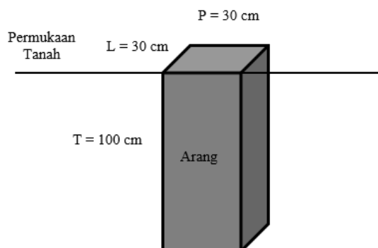
Gambar 3: Ilustrasi Peletakan Arang Aktif pada Sistem Pengetanahan
