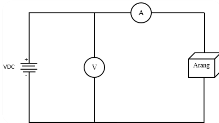
Gambar 4: Rangkaian Pengukuran Tahanan Komposisi Arang Aktif dan Tanah
