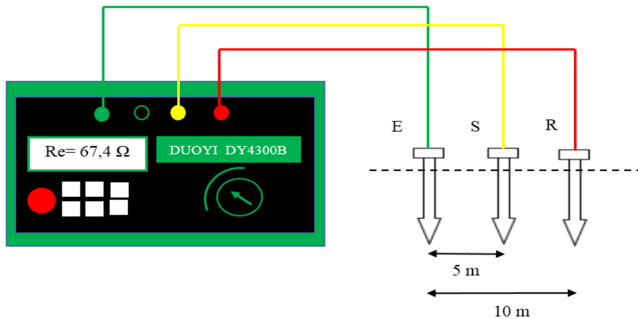
Gambar 5: Rangkaian Pengukuran Tahanan Pengetanahan
